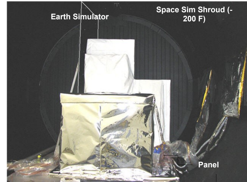
OLI into Space Simulation Chamber
